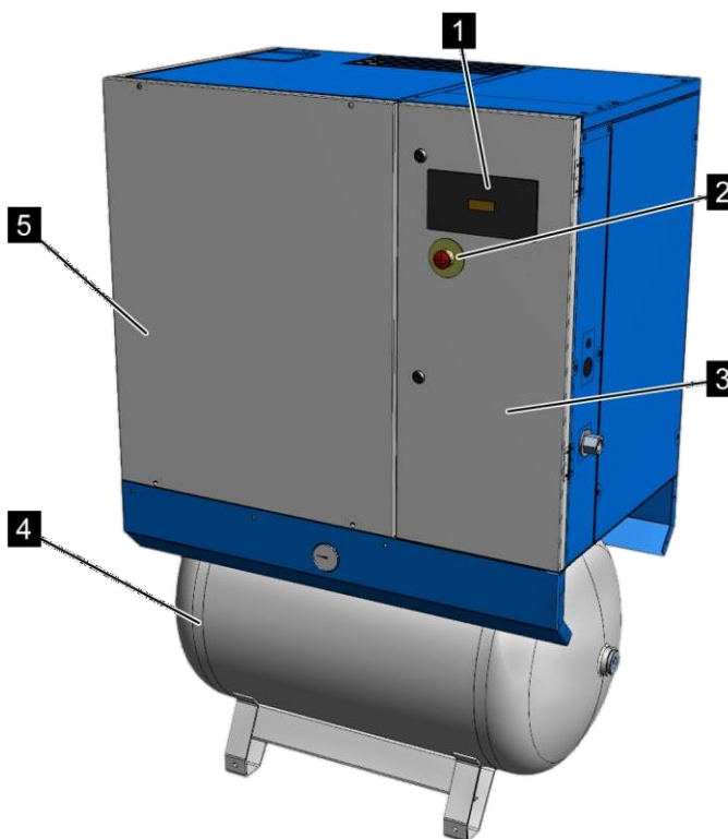
Рис. 8: Винтовой компрессор с баком высокого давления
