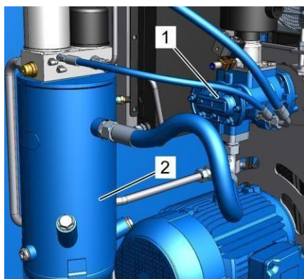
Рис. 17: Ступень компрессора
